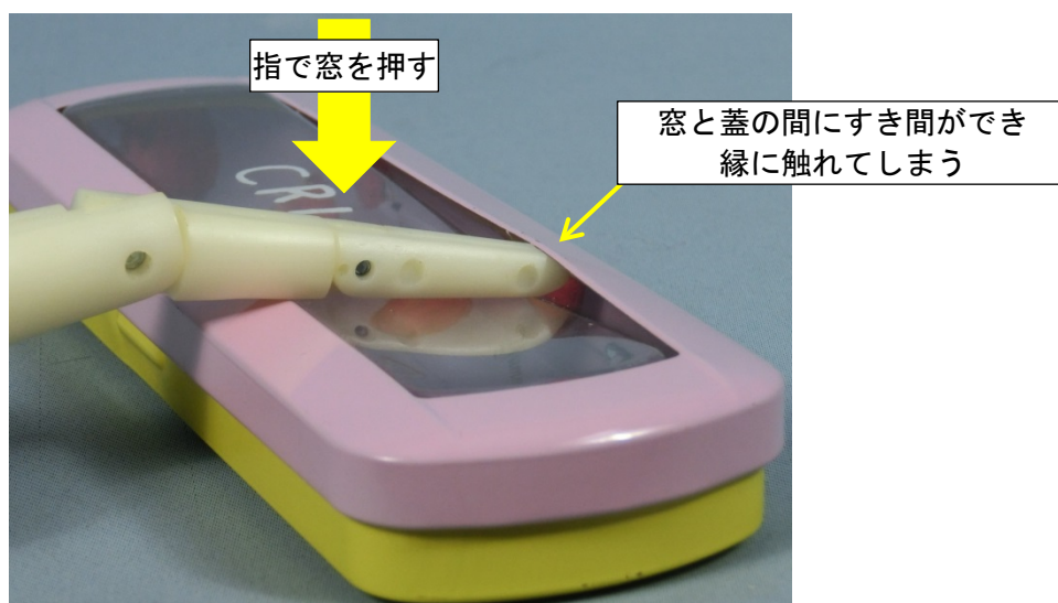
写真3. 窓を指で押すと窓がたわむ様子
